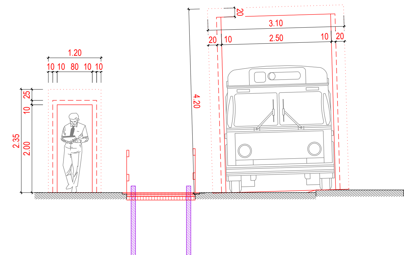
Geometrisches Normalprofil 1:500 V= 30-40 km/h
