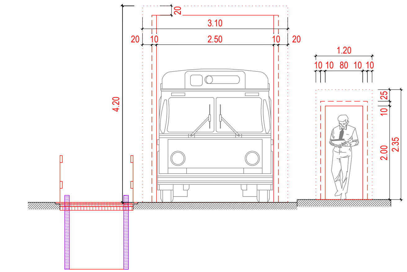
Geometrisches Normalprofil 1:50 V= 30-40 km/h
